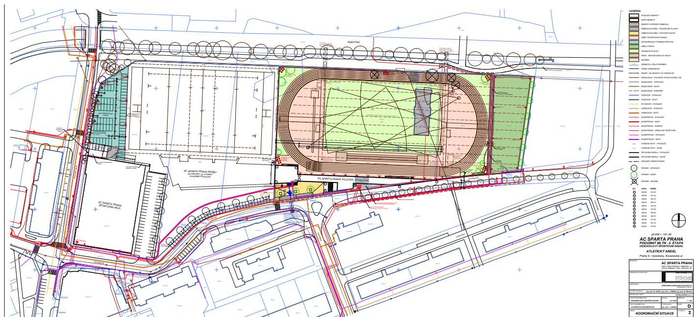
Budoucí podoba venkovního sportovního areálu AC Sparta Praha v Podvíní
